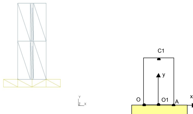
Figure 5.1-a : Modélisation et maillage
