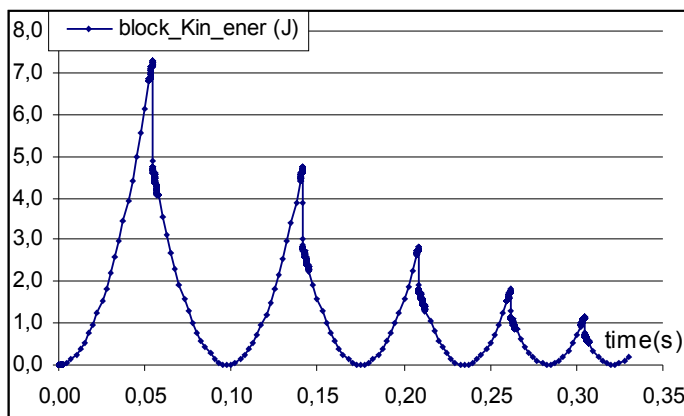
Évolution de l'énergie cinétique (J) du bloc.
