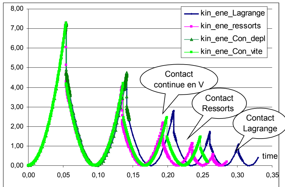
Figure 6-a : Évolution temporelle (temps en s) de l'énergie cinétique (en J ) du bloc selon les méthodes sur machine Bull, avec un schéma d'intégration temporelle implicite en déplacement de type Newmark-HHT (méthode Lagrange ; méthode de pénalisation par ressorts ; méthode continue formulée en déplacement), ou avec un \theta -schéma d'intégration temporelle implicite en déplacement (méthode de contact de type Lagrange).
