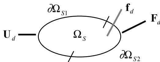
Figure 2.2-2.2-a : Représentation d'un problème de calcul de structure
