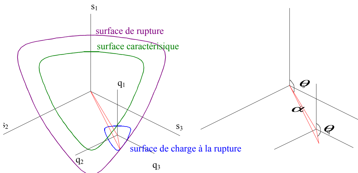
Figure 3.4.4-a : Représentation des surfaces de rupture, caractéristique et de charge dans le plan déviateur
