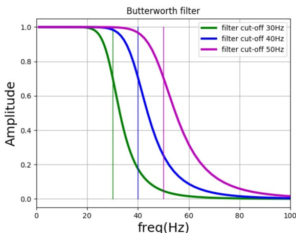
Figure 1 : illustration de l'allure du filtre de Butterworth pour différentes fréquences de coupure
